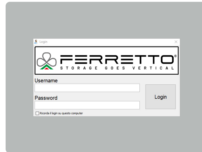
Login page
